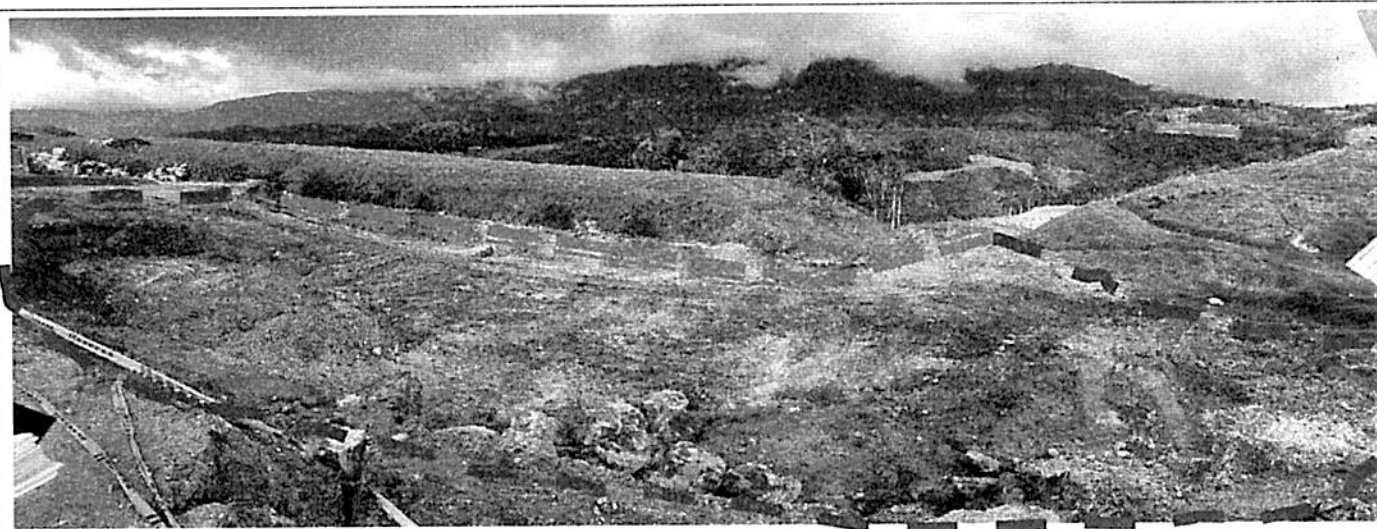
Fotografía 5. Panorámica de la zona donde se ejecuta el proyecto de optimización del relleno sanitario "La Cortada" en Pamplona, Fase II. Se observan labores de excavación en la zona norte. Las líneas azules señalan el alineamiento del muro de contención en tierra armada y el rojo el contorno aproximado del vaso de disposición final costado norte.
