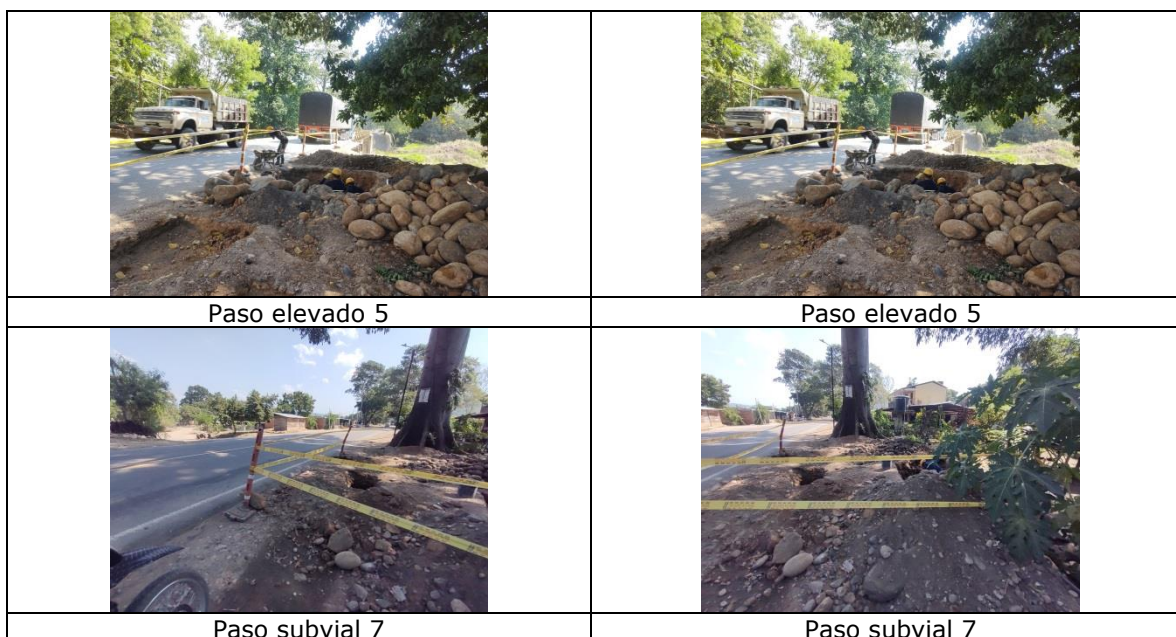
Figura. Construcción paso elevado 5 y paso subvial 7
